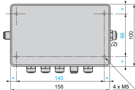
XGSZ33PDP (PROFIBUS DP) and XGSZ33EIP (EtherNet/IP) boxes
