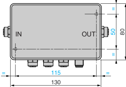
XGSZ33PDP (PROFIBUS DP) and XGSZ33EIP (EtherNet/IP) boxes
