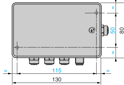
XGSZ33ETH (Ethernet) box
